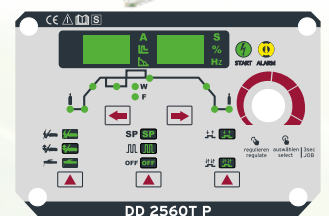
Bedienpanel DD 2560T P
